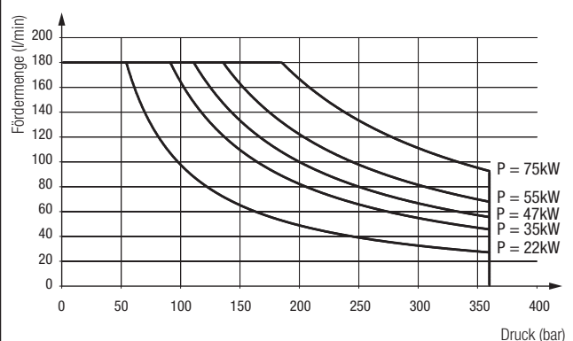
Beispiel: Fördermenge kennzeichnende Kurve
