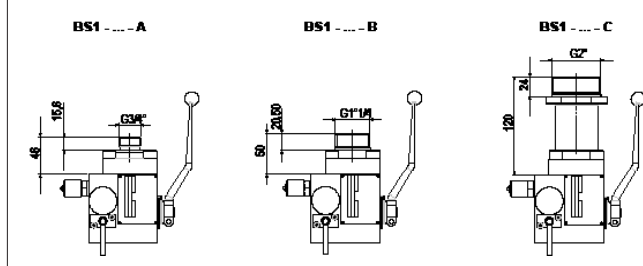
Flansch für Sicherheitsblöcke BS1.
