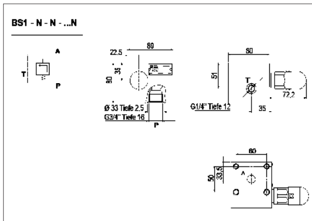
Flansch für Sicherheitsblöcke BS1.
