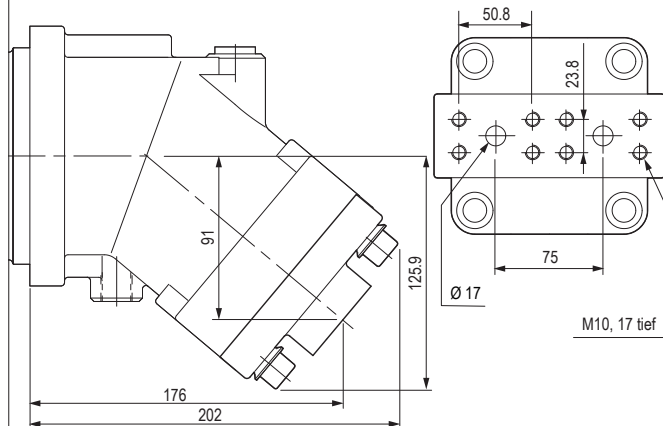
P0 Gewindeanschlüsse hinten
