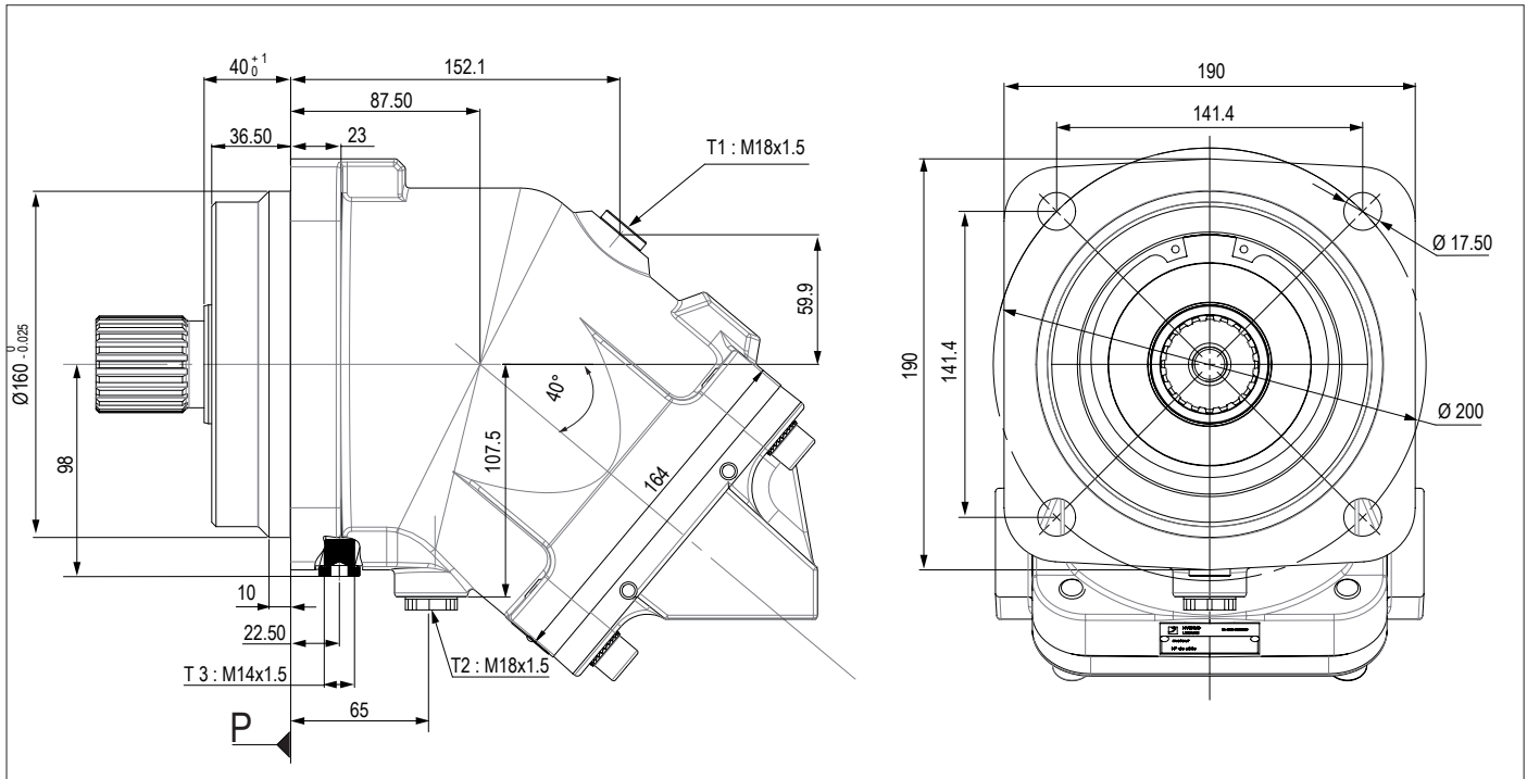
W1 Zahnwelle DIN 5480 W 45 x 2 x 30 x 21 x 9 g
