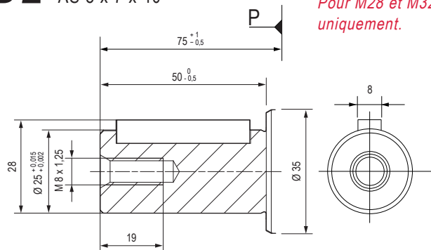
D2 Axe Ø 25 cylindrique à clavette DIN 6885 AS 8 x 7 x 40 Pour M28 et M32 uniquement.
